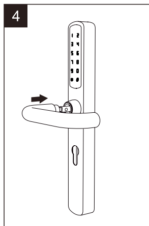
4. Nasad'te kliku zpět na čtyřhran
