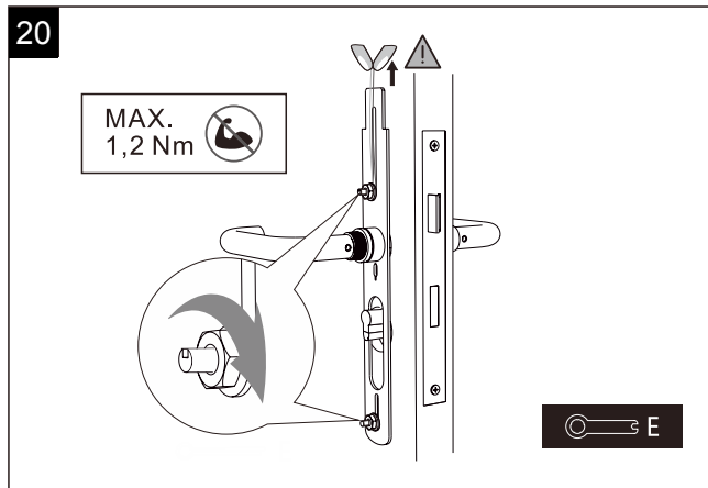
20. Nyní dotáhněte matice speciálním stranovým klíčem (matice „neutahujte“ přílišnou silou)
