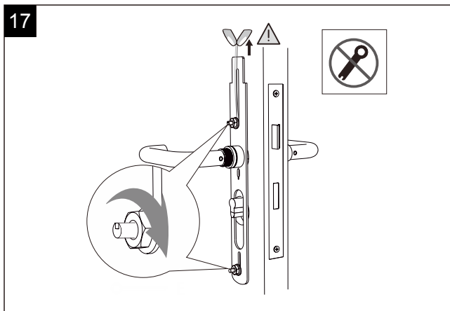
17. Dotáhněte matici rukou, zatím bez použití stranového klíče
