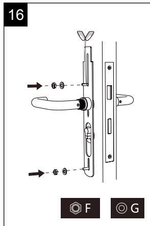
16. Namontujte podložku a matici
